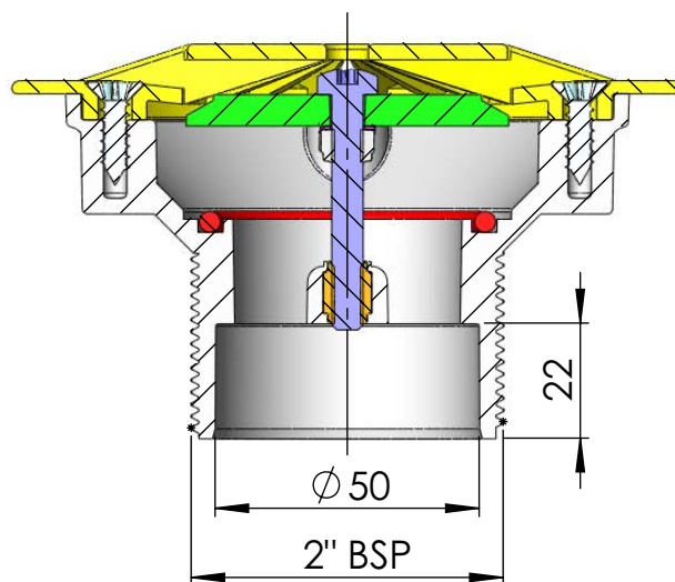
SECCIÓN B-B
